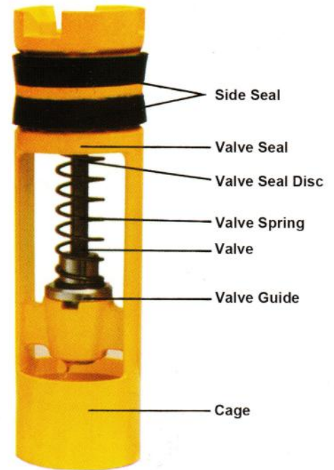
Piston Type
